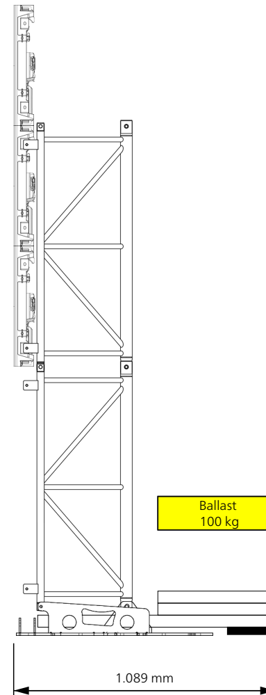
Seitenansicht
