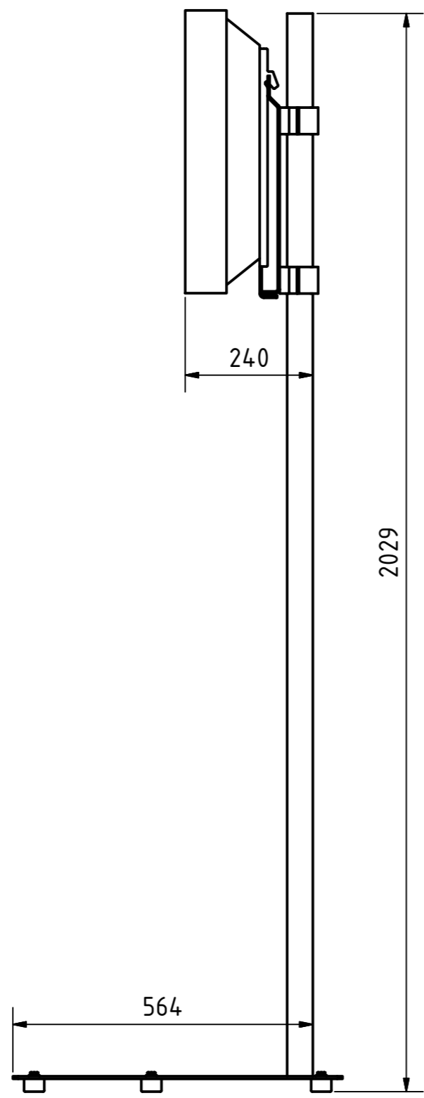
Rechts ( 1 : 10 )
