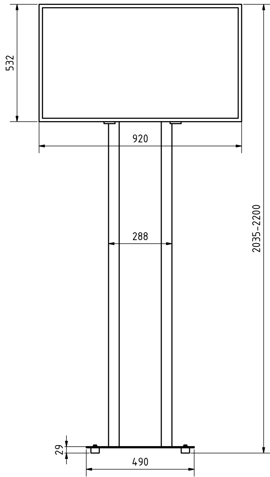
Vorne ( 1 : 10 )
