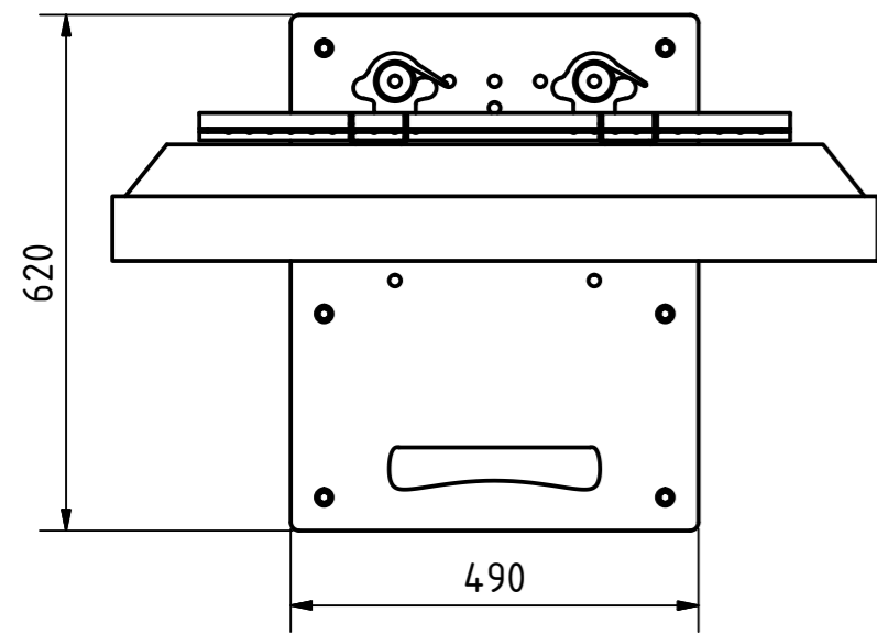
Oben ( 1 : 10 )
